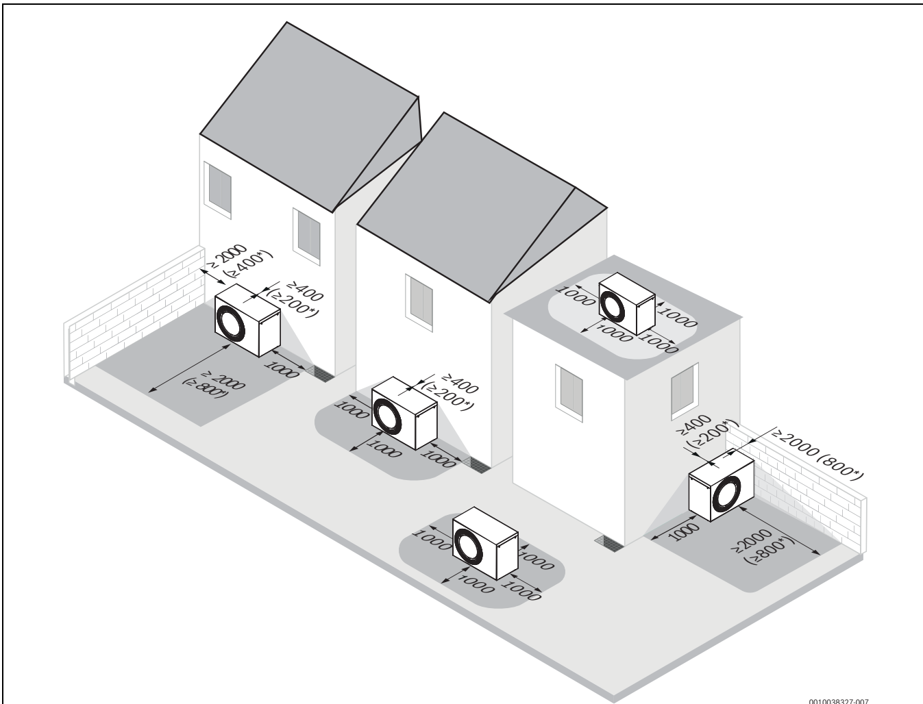
Bild 23 Empfohlener Abstand zwischen der Wärmepumpe und umgebenden festen Objekten (mm)
