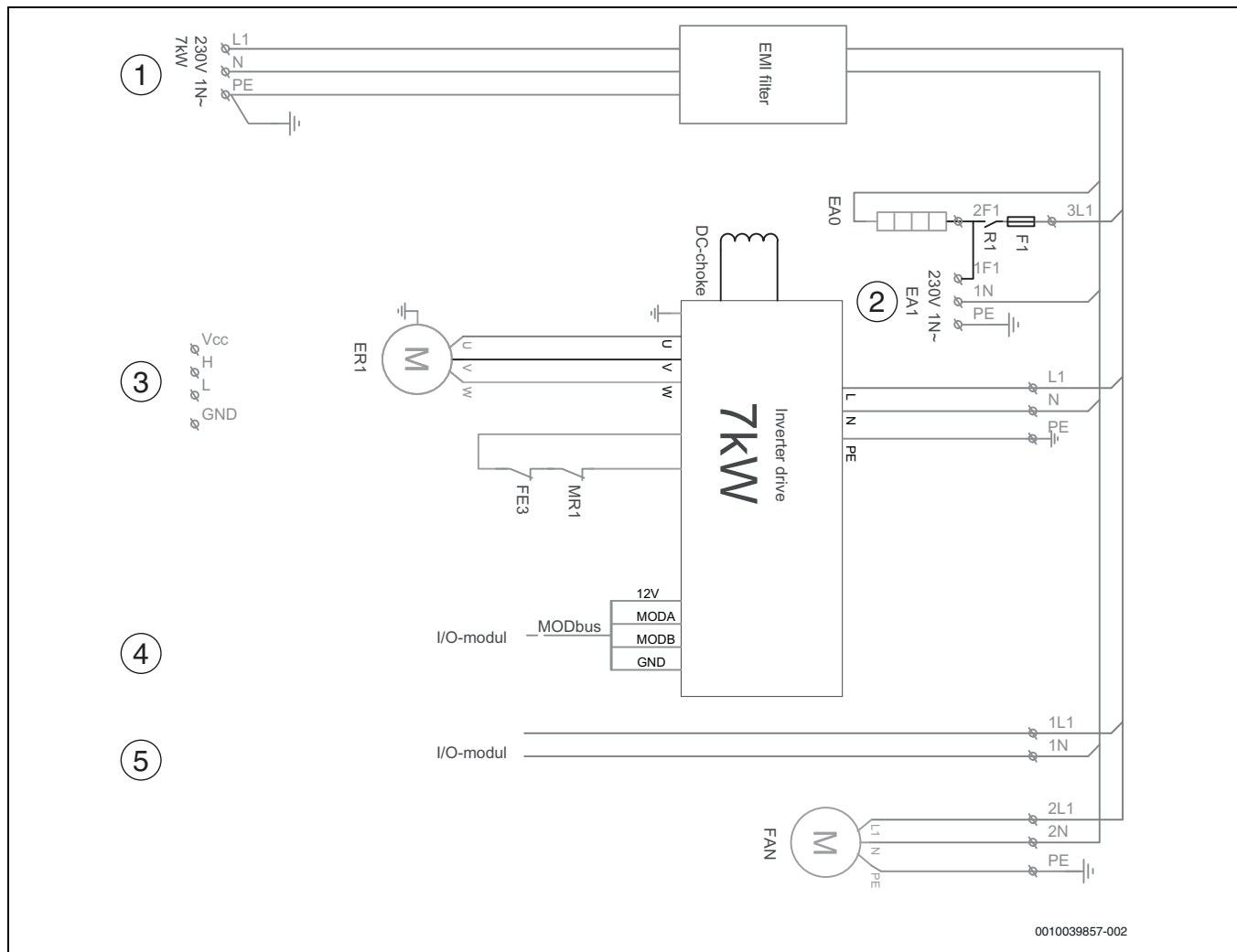
Bild 54 Schaltplan Frequenzumrichter
