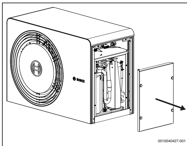
Bild 39 Abdeckung der Kältekreisbox
