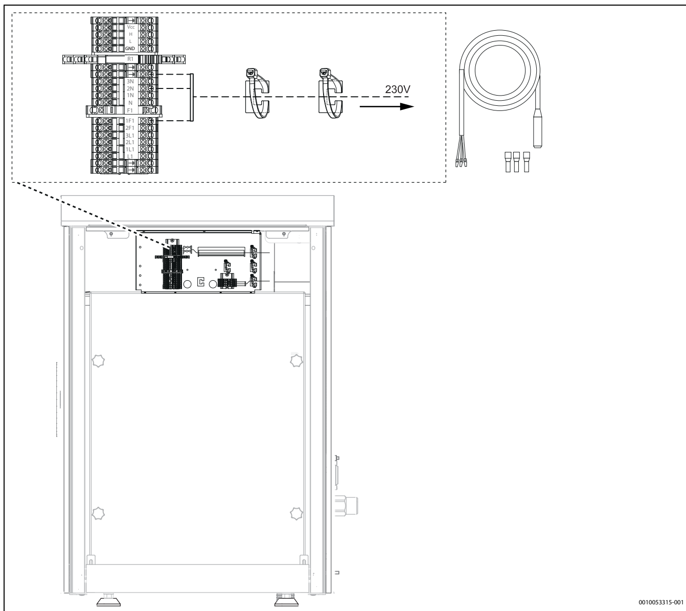
Bild 46 Heizkabelanschluss (Zubehör)
