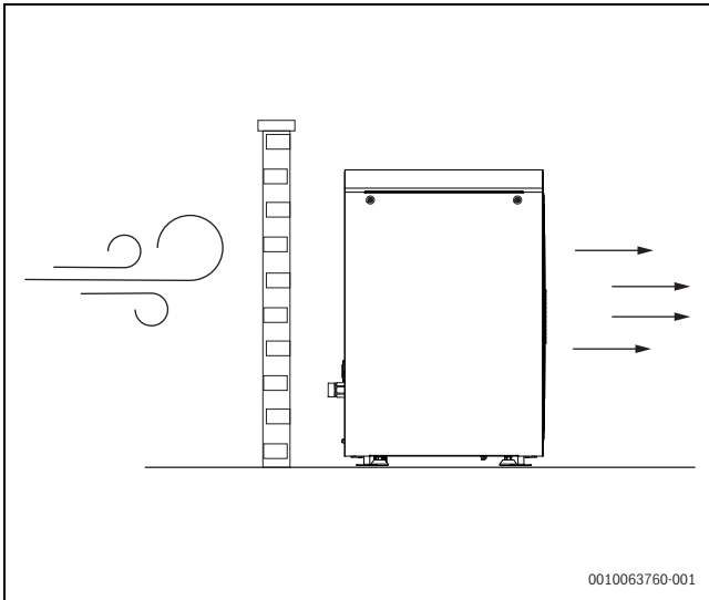
Bild 22 Freistehende Wärmepumpe
