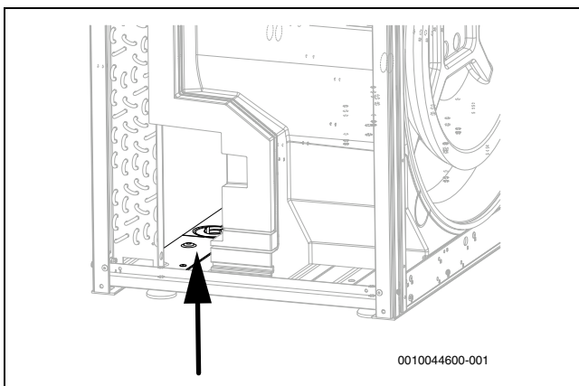
Bild 49 Auffangwanne reinigen
