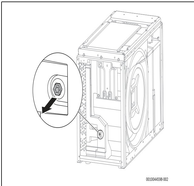
Bild 47 Abschrauben
