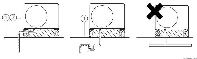
Bild 34 Kondensatableitung in die Kanalisation/Regenwasserablauf
