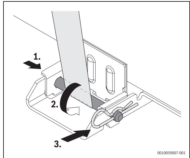
Bild 18 Einstecken von Verschlussleiste, Stift und Gurt
