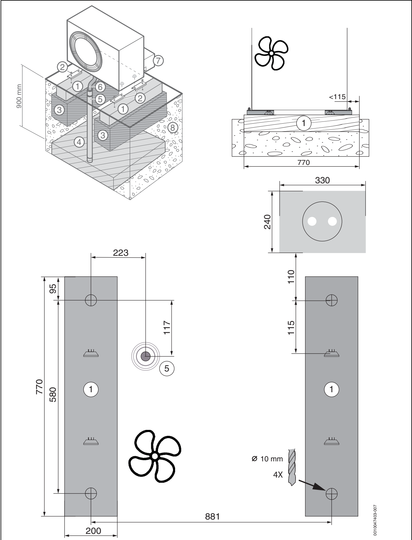
Bild 35 Fundamentplan, Alternative 1
