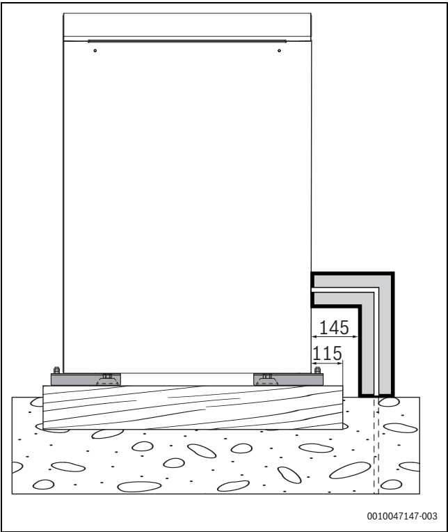
Bild 28 Montageset, Seitenansicht
