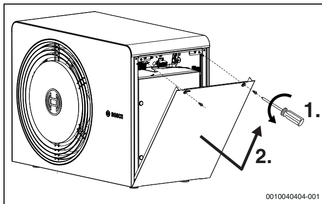
Bild 38 Seitliche Abdeckung
