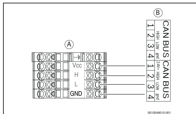
Bild 41 CAN-BUS Wärmepumpe - Inneneinheit
