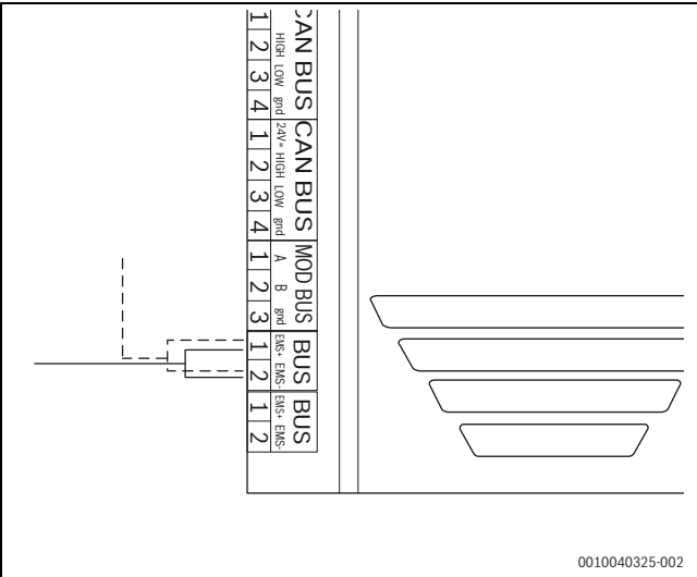
Fig. 11 Collegamento EMS
