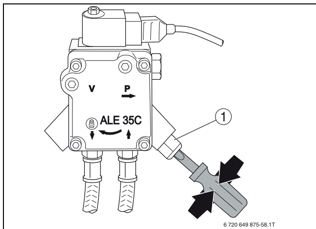
Fig. 27 Impostazione della pressione – pompa gasolio Suntec
