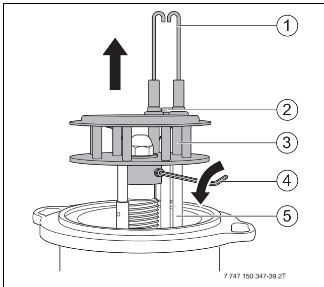
Fig. 37 Smontaggio del sistema di miscelazione
