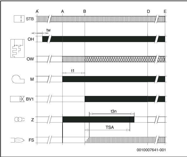
Fig. 7 Svolgimento del programma dell'automatismo di combustione
