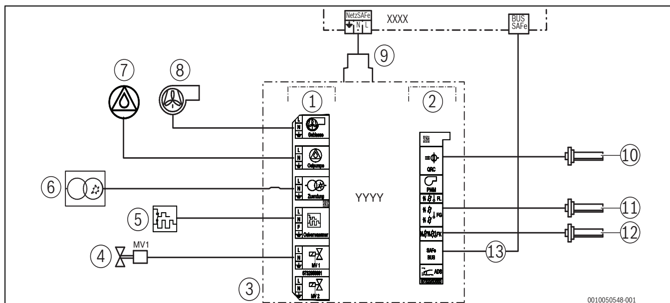
Fig. 10 Schema elettrico di collegamento automatismo digitale di combustione SAFe100
