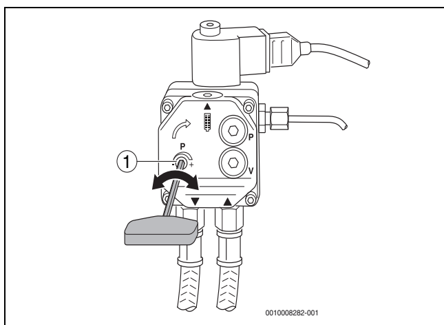
Fig. 26 Impostazione della pressione – pompa gasolio Danfoss
