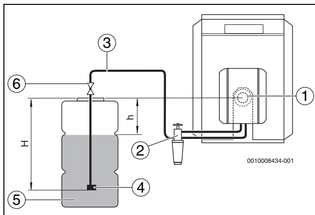
Fig. 14 Serbatoio del gasolio sotto la pompa
