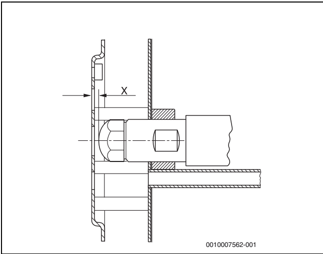
Fig. 4 Sistema di miscelazione – Misura "X"
