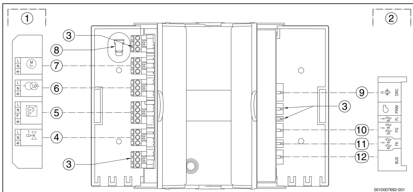
Fig. 9 Schema elettrico di collegamento automatismo digitale di combustione SAFe30
