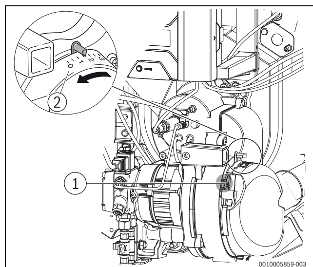
Fig. 25 Impostazione del carter di aspirazione dell'aria
