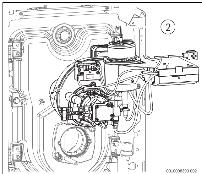
Fig. 36 Posizionare il bruciatore in posizione di servizio
