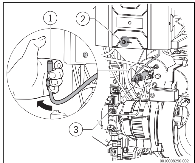
Fig. 44 Verifica del funzionamento della fotocellula
