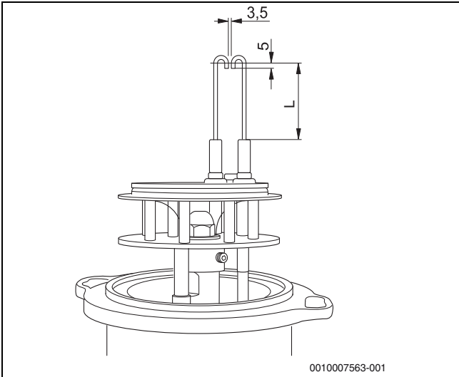
Fig. 3 Elettrodo di accensione (dimensioni in mm)
