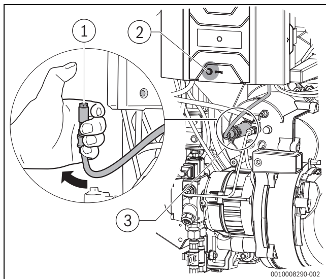
Fig. 28 Verifica del funzionamento della fotocellula
