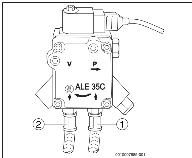
Fig. 17 Pompa gasolio – Suntec
