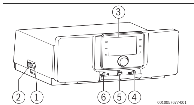
Fig. 19 Unità di termoregolazione con termoregolatore
