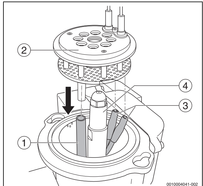
Fig. 39 Montaggio del sistema di miscelazione
