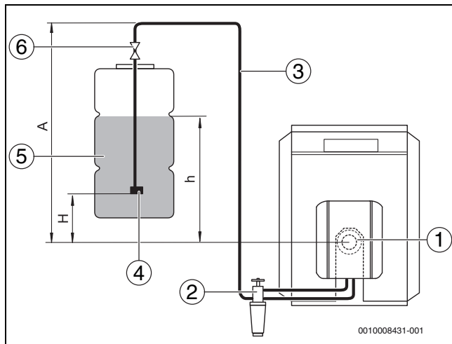
Fig. 13 Serbatoio del gasolio sopra la pompa
