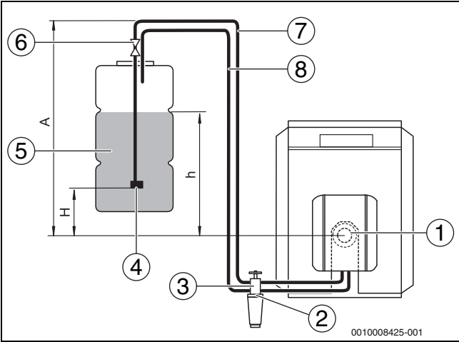
Fig. 11 Serbatoio del gasolio sopra la pompa
