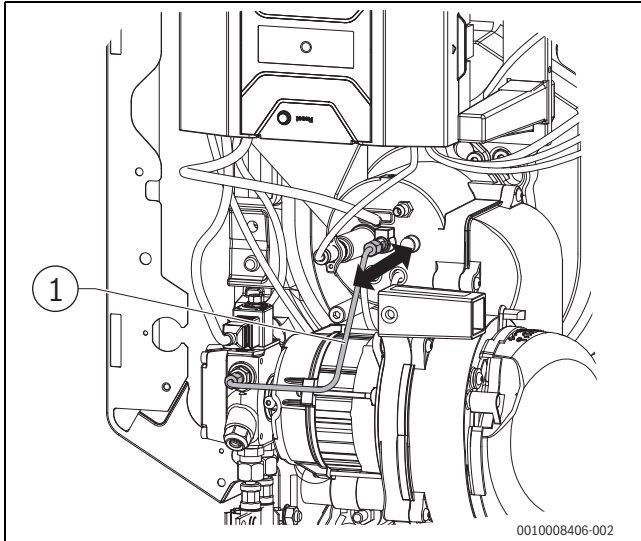
Fig. 42 Verifica della posizione corretta del sistema di miscelazione
