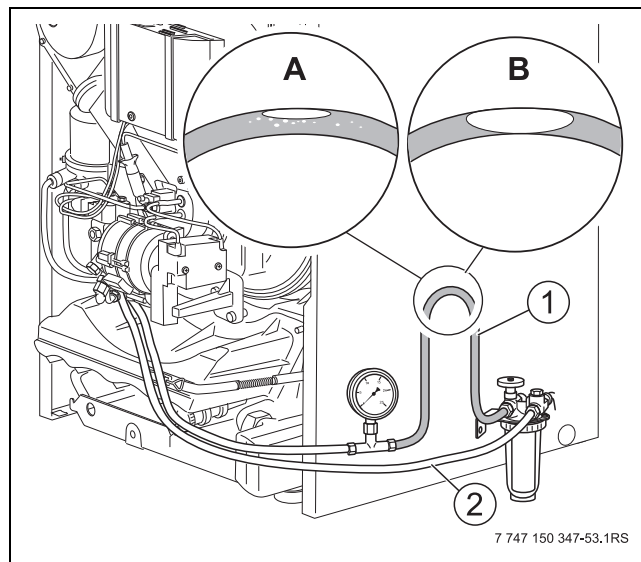
Fig. 15 Legare in alto il tubo flessibile trasparente
