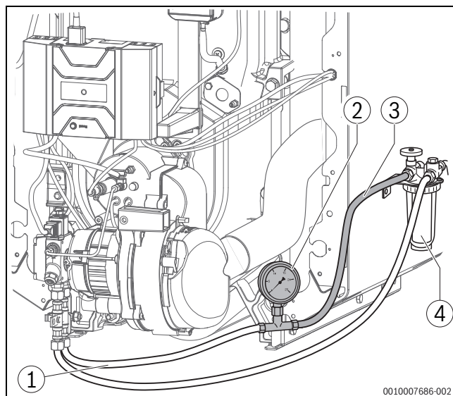
Fig. 18 Filtro del gasolio, vacuometro e flessibile trasparente (illustrati: 18-49 kW)
