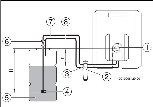
Fig. 12 Serbatoio del gasolio sotto la pompa
