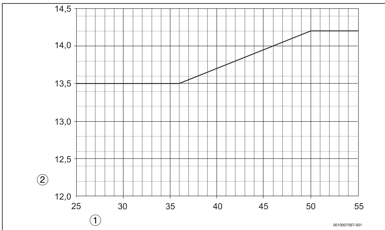
Fig. 24 Impostazione del tenore di CO 2 con aspirazione dell'aria di alimentazione tramite sistema concentrico di aspirazione e scarico gas combusti (funzionamento con flessibile di aspirazione)
