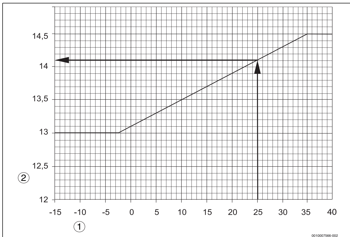
Fig. 23 Impostazione del tenore di CO 2 con aspirazione dell'aria di alimentazione attraverso la parete esterna (funzionamento con flessibile di aspirazione)
