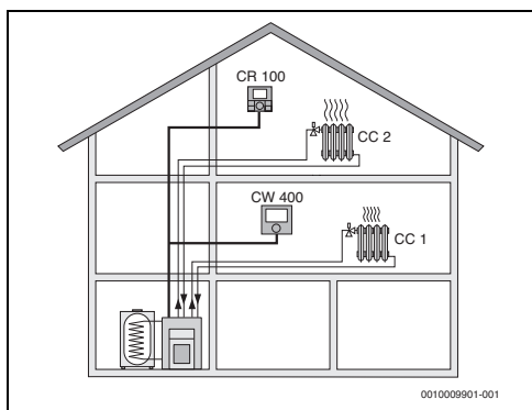
Fig. 2 CR 100 en tant que commande à distance pour le deuxième circuit de chauffage (CC 2) et C 400/C 800 en tant que régulateur pour le premier circuit (CC 1)
