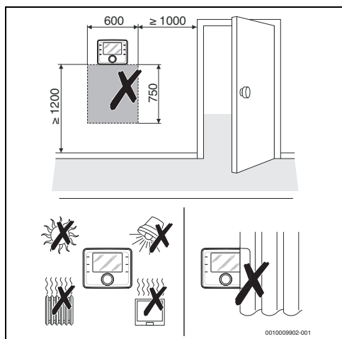
Fig. 5 Lieu d'installation dans la pièce de référence
