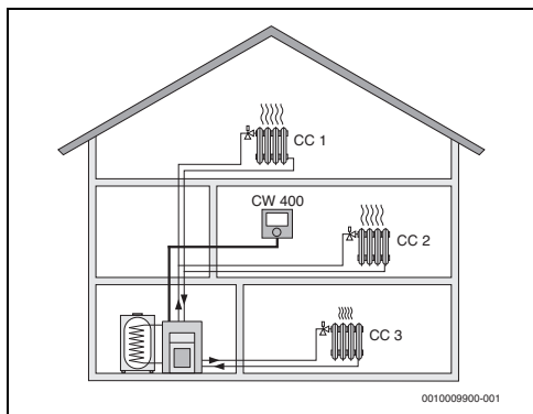
Fig. 1 C 400/C 800 en tant que régulateur pour plusieurs (dans ce cas trois) circuits de chauffage
