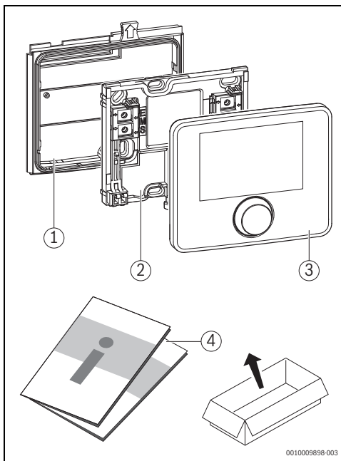
Fig. 3 Contenu de la livraison
