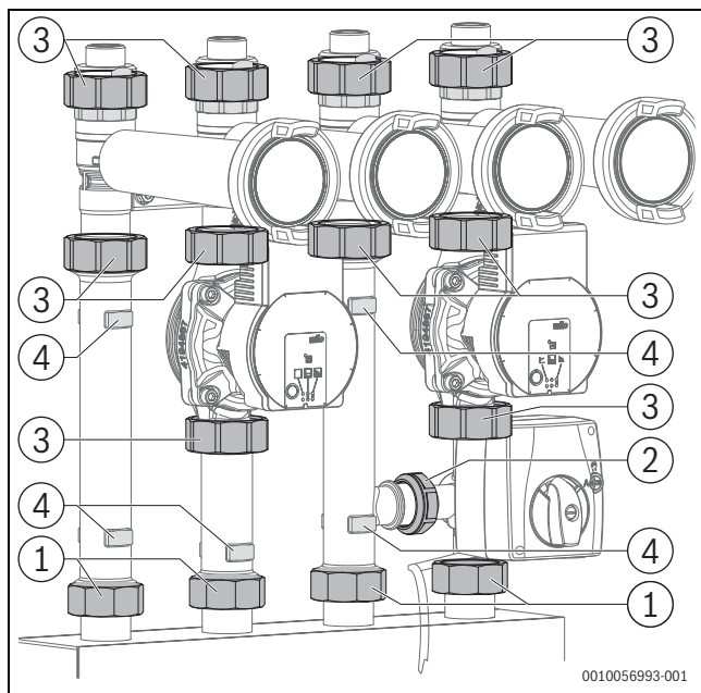
Fig. 13 Dadi a risvolto e superfici di presa (esempio: circuito riscaldamento misto)
