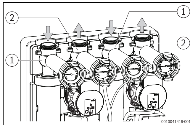
Fig. 24 Rubinetti a sfera
