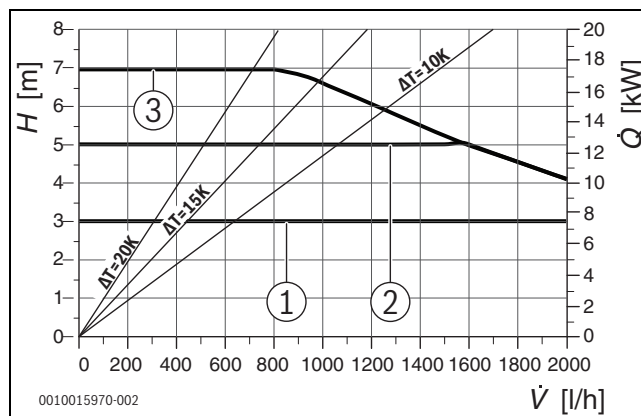
Fig. 7 Curve caratteristiche circolatore pressione differenziale costante
