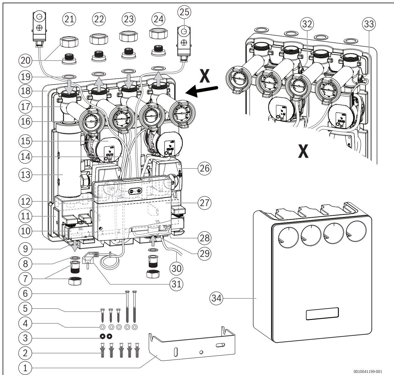
Fig. 9 Panoramica del prodotto HSM2-M 20/7 MM200
