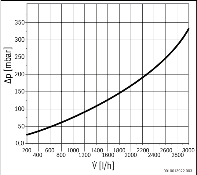
Fig. 12 Diagramma perdita di carico circuito di riscaldamento diretto
