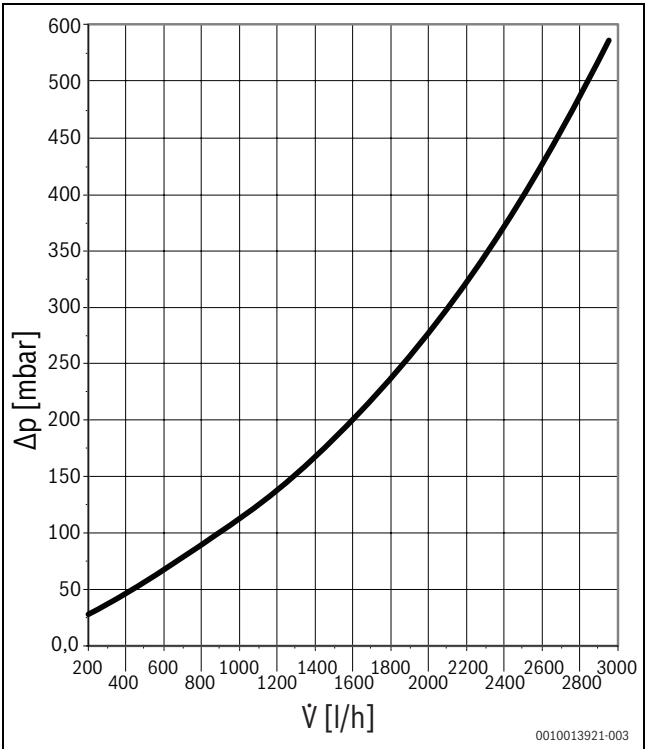
Fig. 11 Diagramma perdita di carico circuito di riscaldamento miscelato
