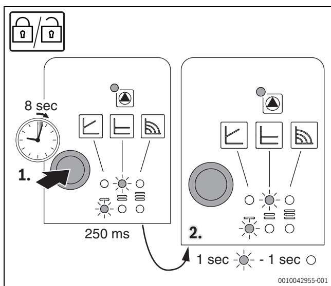
Fig. 30 Impostazione del circolatore, tasto blocco/sblocco
