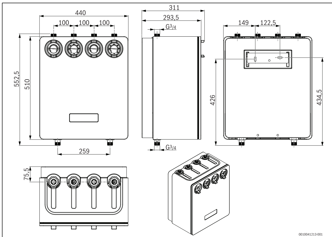
Fig. 10 Dimensioni e collegamenti (misure in mm)
