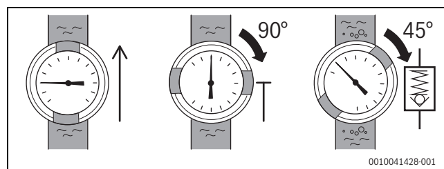
Fig. 25 Impostazioni dei rubinetti a sfera, mandata
