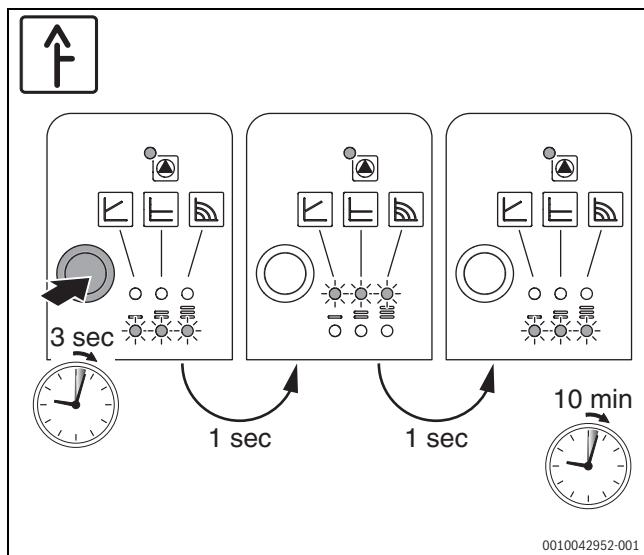
Fig. 28 Impostazione del circolatore, sfiato
