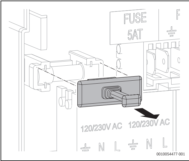
Fig. 32 Sostituire il fusibile
