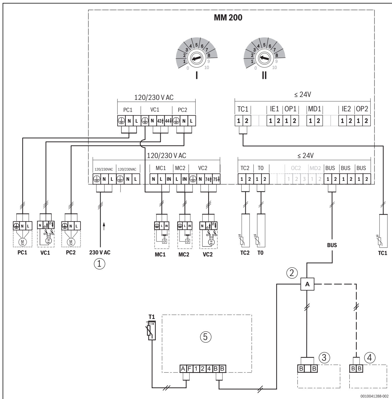
Fig. 23 Schema elettrico di collegamento HSM2-M 20/7 MM200
