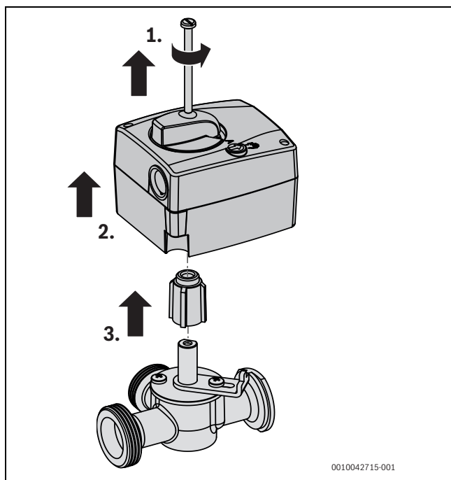
Fig. 34 Rimozione del motore valvola miscelatrice
