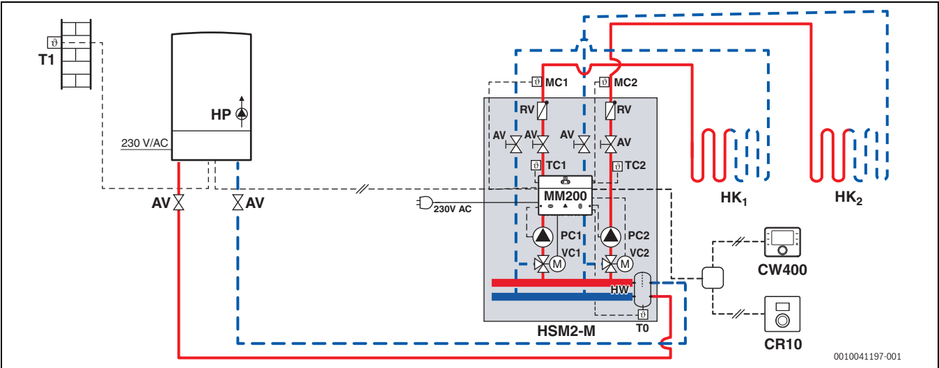
Fig. 2 Esempio di impiego HSM2-M 20/7 MM200
