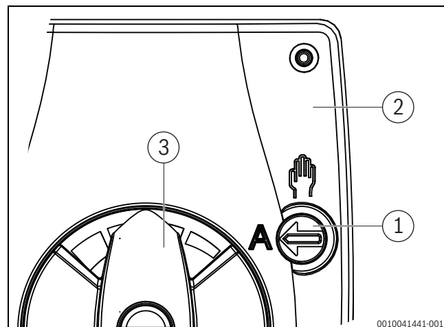
Fig. 31 Motore valvola miscelatrice
