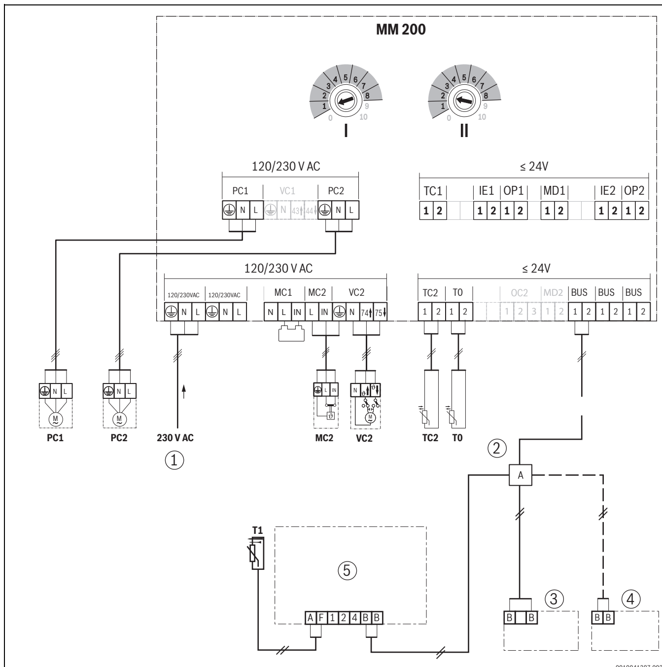
Fig. 22 Schema elettrico di collegamento HSM2-U 20/7 MM200
