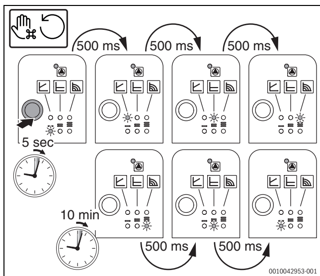
Fig. 29 Impostazione del circolatore, riavvio manuale
