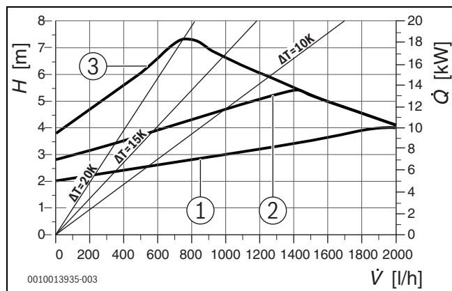
Fig. 6 Curve caratteristiche circolatore pressione differenziale variabile
