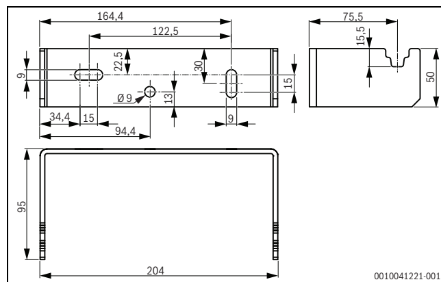
Fig. 14 Dimensioni del supporto a parete
