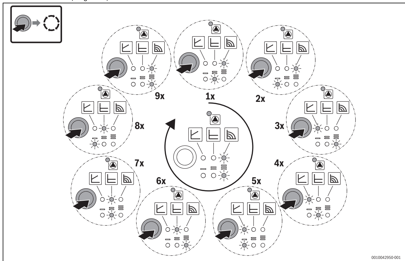
Fig. 27 Impostazione del circolatore, modalità di regolazione e curve caratteristiche
