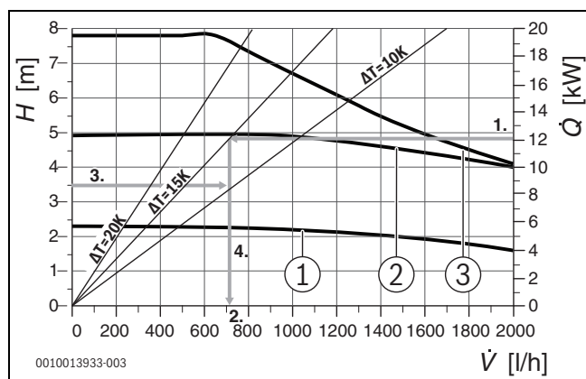
Fig. 5 Curve caratteristiche pompe con velocità costante
