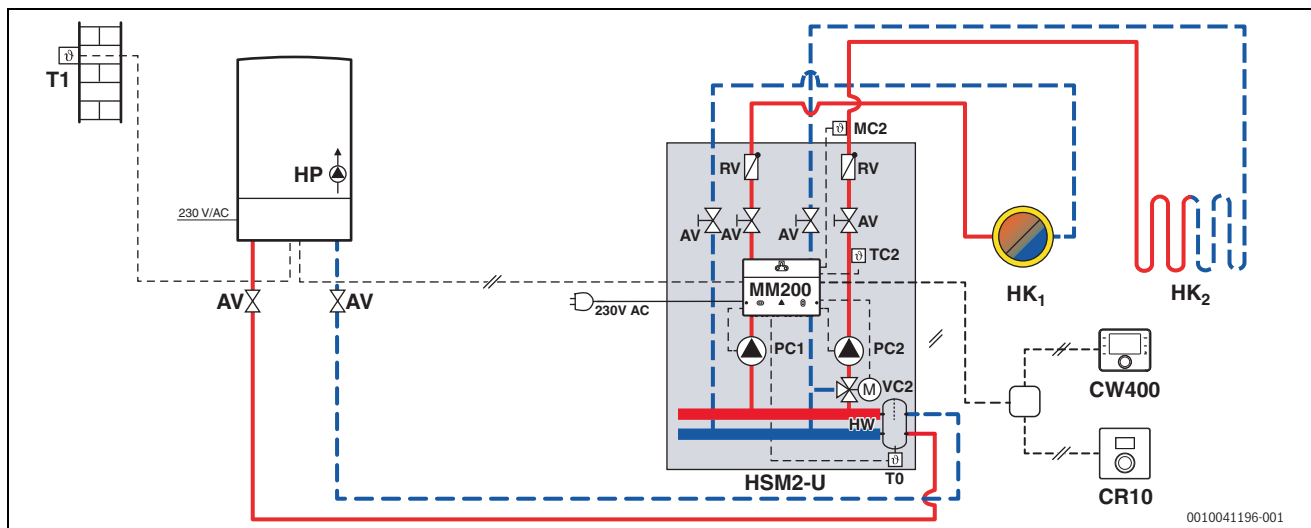
Fig. 1 Esempio di impiego HSM2-U 20/7 MM200
