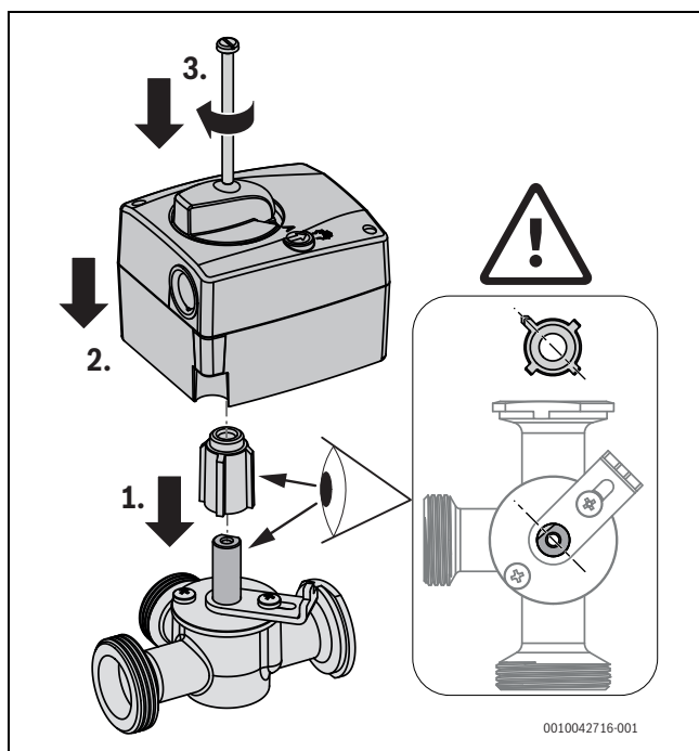
Fig. 35 Installazione del motore valvola miscelatrice
