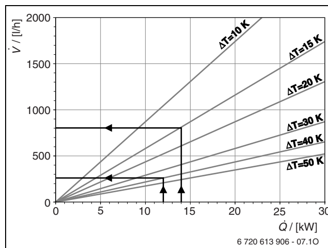
Fig. 4 Potenza termica in funzione della portata
