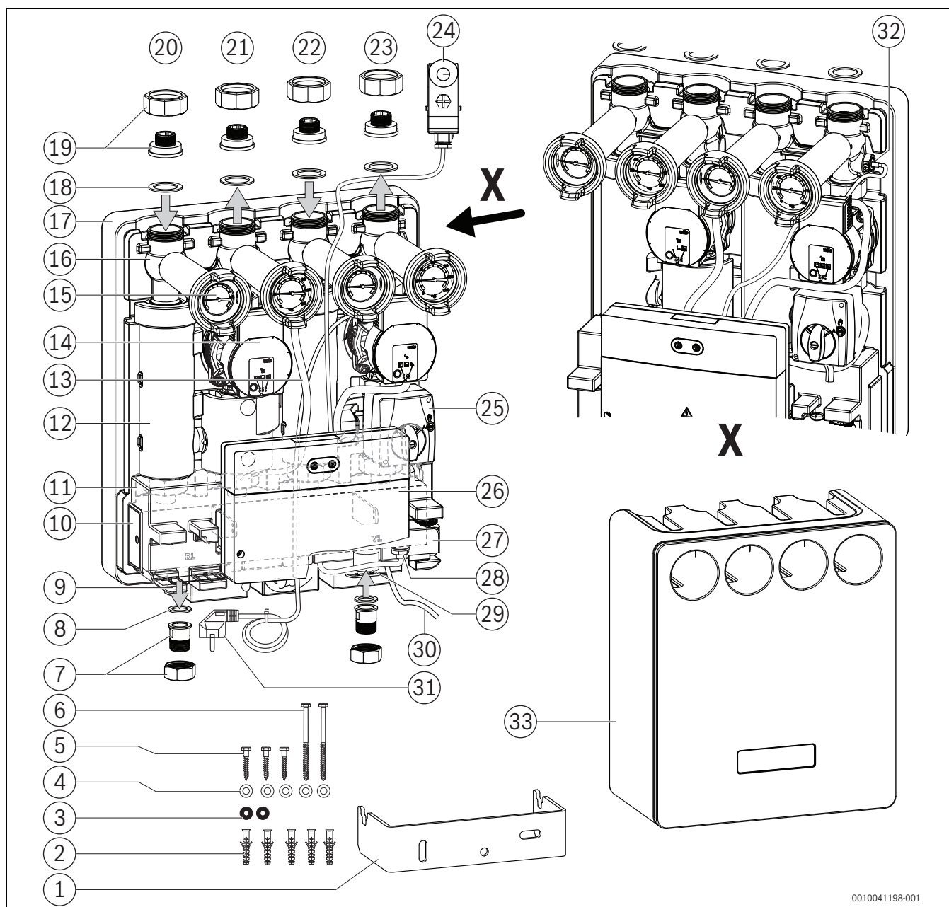
Fig. 8 Panoramica del prodotto HSM2-U 20/7 MM200
