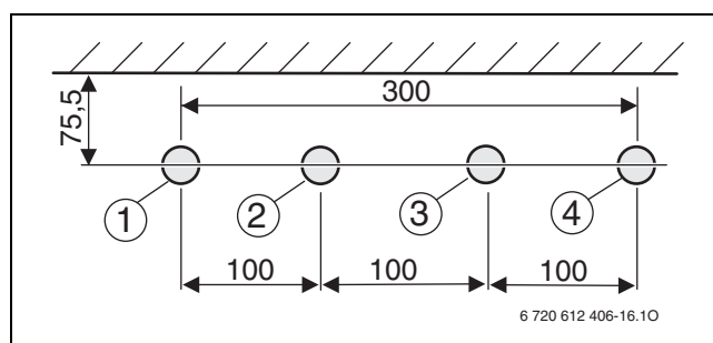
Fig. 17 Misure per l'installazione dei collegamenti da parte del committente
