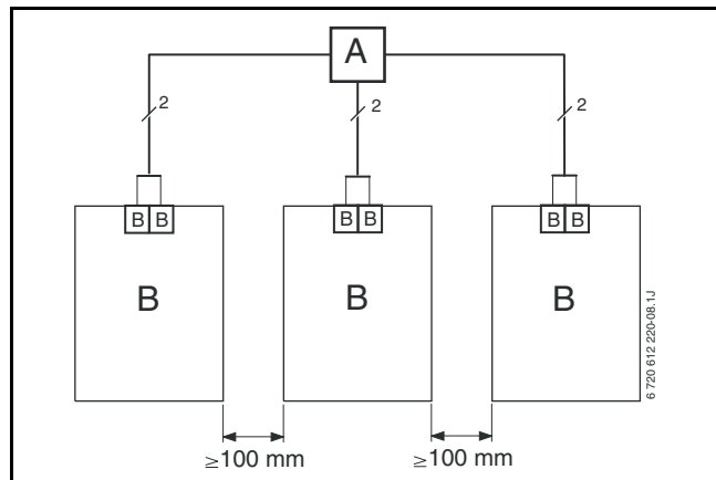
Fig. 21 Collegamento dei cavi BUS con scatola di derivazione (A)
