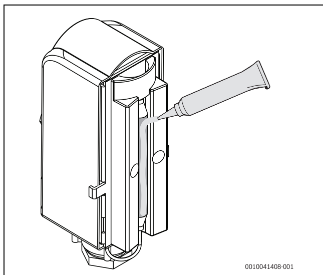
Fig. 18 Applicazione della pasta termoconduttrice
