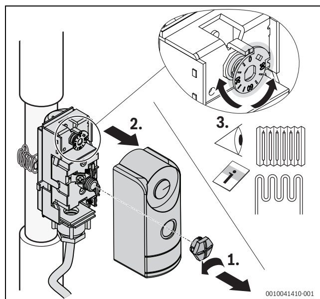
Fig. 20 Impostazione della temperatura
