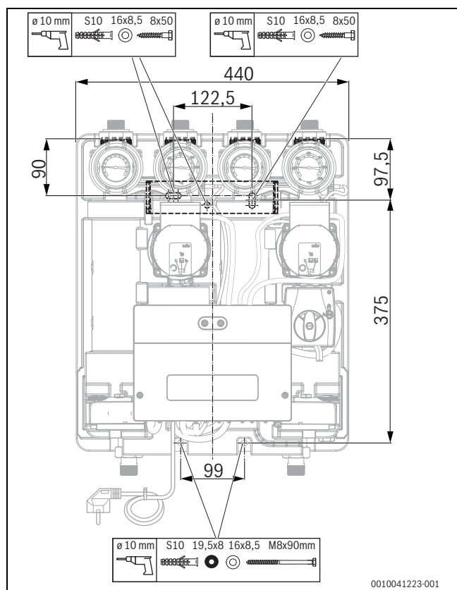
Fig. 15 Fissaggio alla parete sull'esempio del modulo HSM2-M 20/7 MM200
