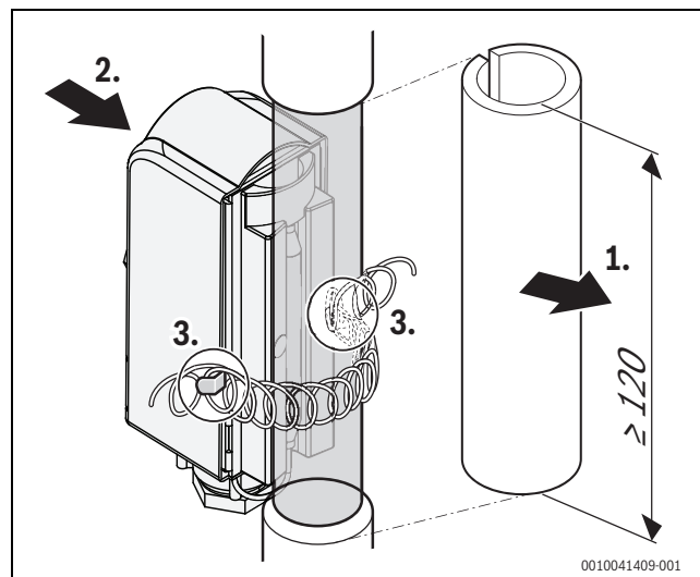
Fig. 19 Installazione del termostato di sicurezza
