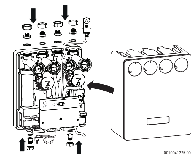
Fig. 16 Installazione dell'isolamento termico
