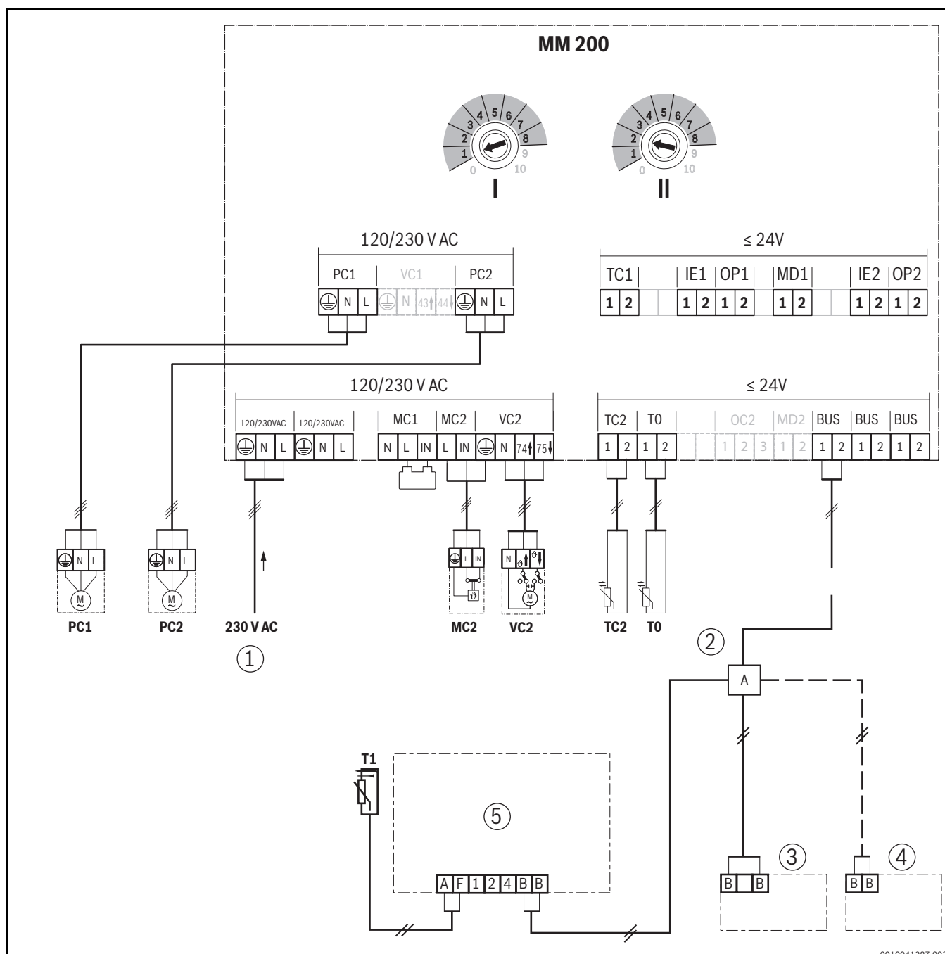
Bild 22 Anschlussplan HSM2-U 20/7 MM200
