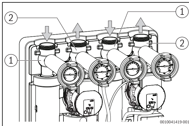
Bild 24 Kugelhähne
