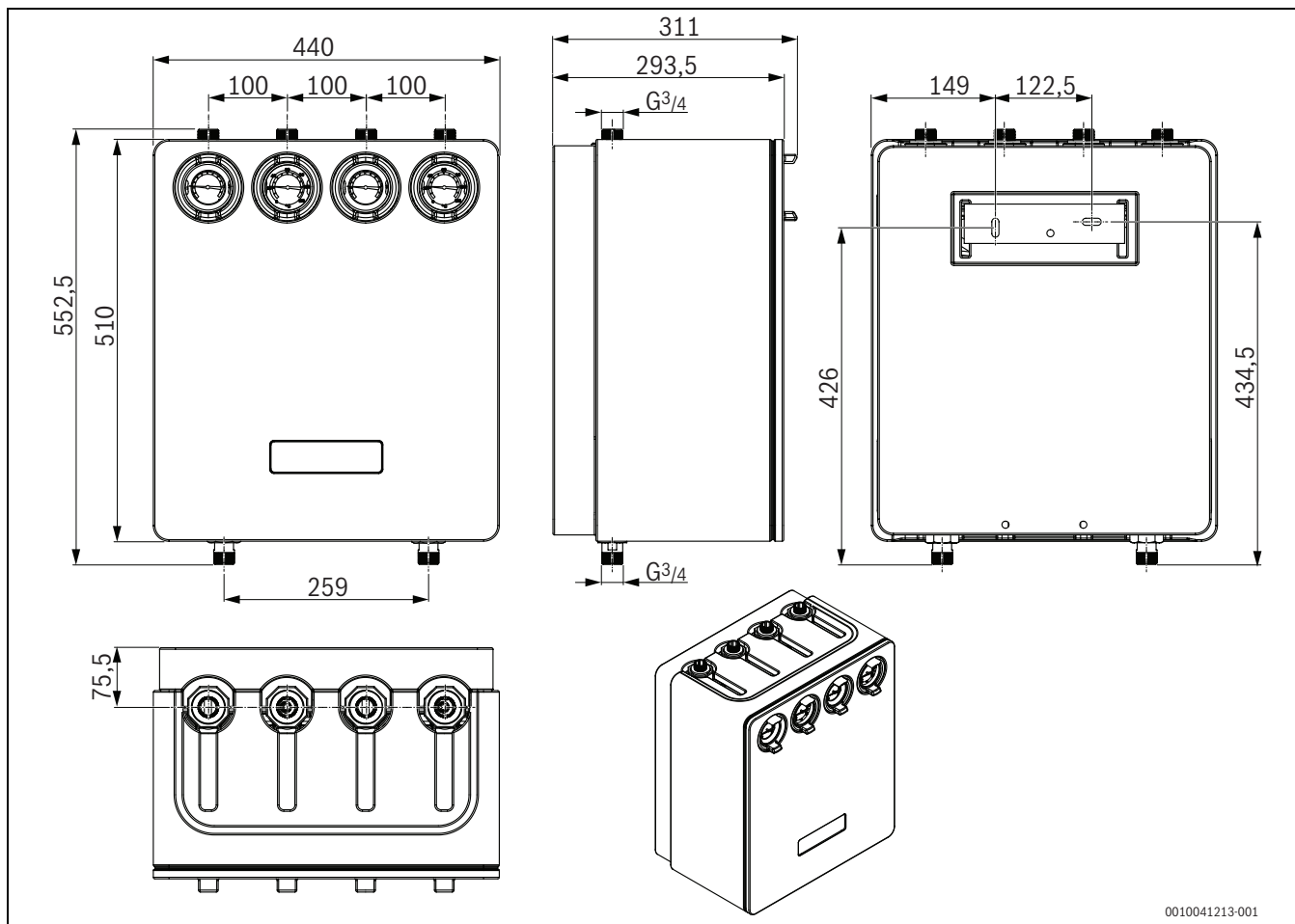
Bild 10 Abmessungen und Anschlüsse (Maße in mm)
