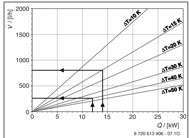
Bild 4 Volumenstrom-Wärmeleistung
