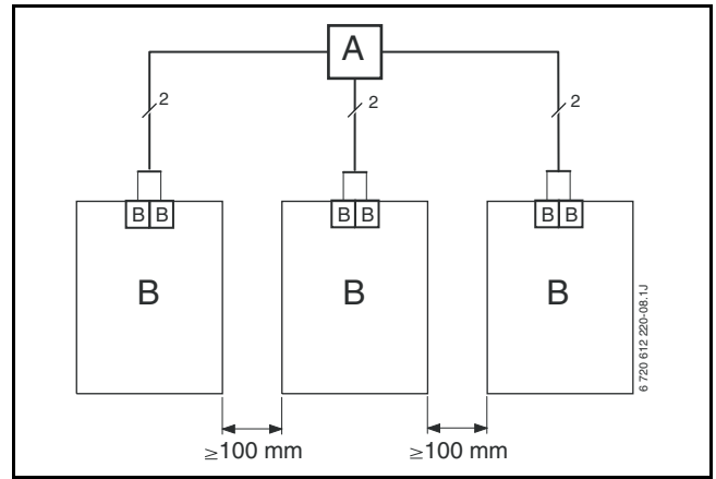
Bild 21 Anschluss der BUS-Leitungen über Verteilerdose (A)
