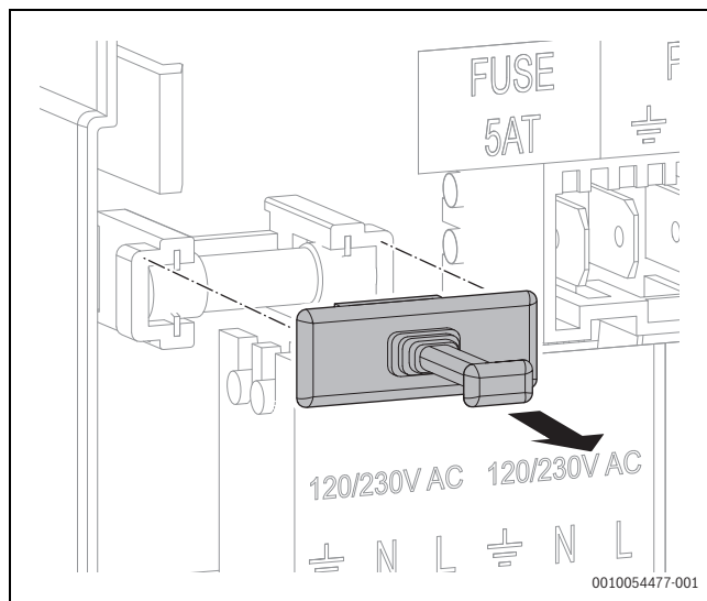
Bild 32 Sicherung tauschen
