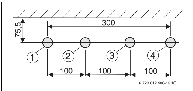
Bild 17 Maße für bauseitige Anschlussinstallation
