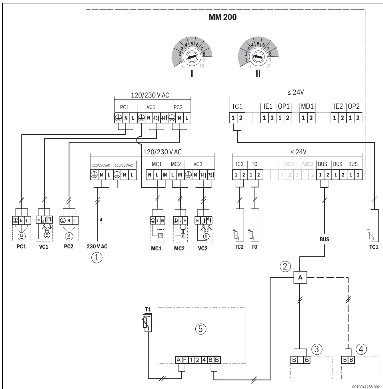
Bild 23 Anschlussplan HSM2-M 20/7 MM200
