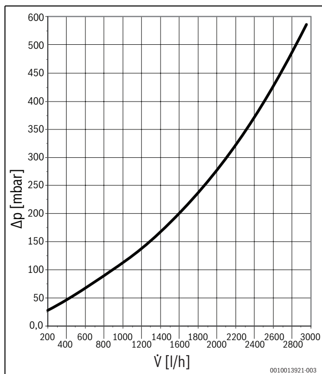
Bild 11 Druckverlust-Diagramm gemischter Heizkreis
