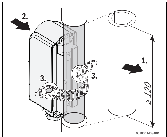
Bild 19 Temperaturwächter montieren
