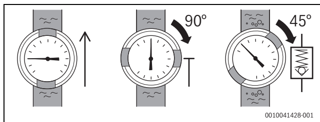
Bild 25 Einstellungen der Kugelhähne, Vorlauf
