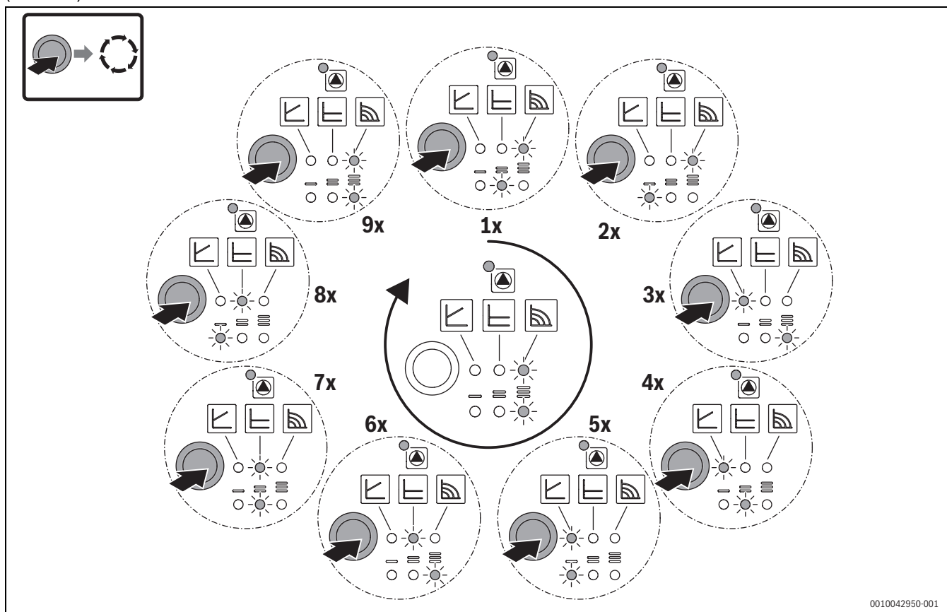
Bild 27 Einstellung der Pumpe, Regelungsart und Kennlinien
