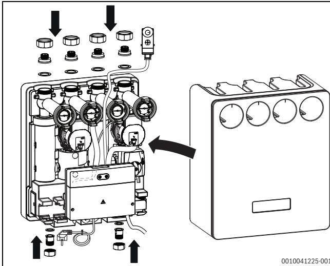
Bild 16 Montage Wärmeschutz
