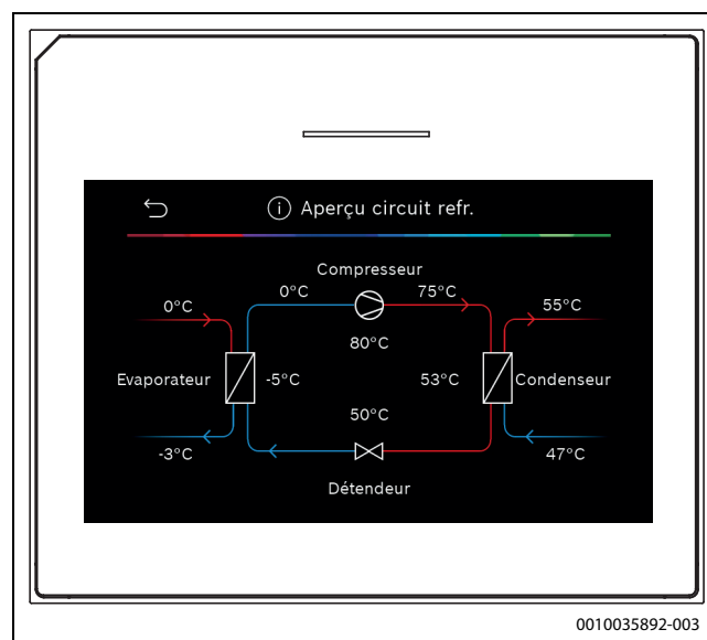
Fig. 10 Aperçu du circuit frigorifique
