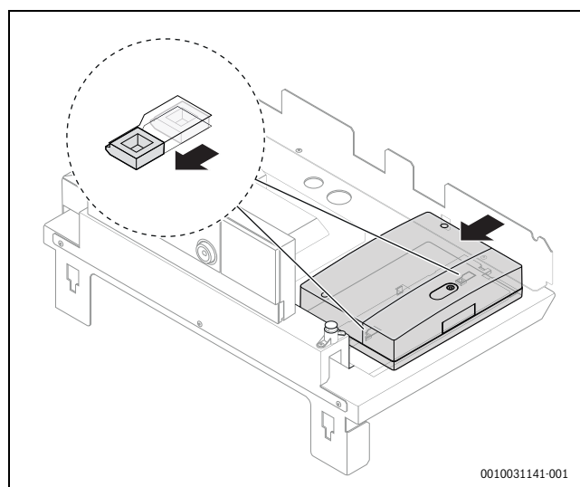
Fig. 18 Montage du module électronique sous le capot de la chaudière (exemple)
