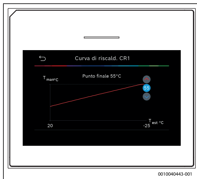
Fig. 2 Regolare il punto finale (solo se si è impostato il tipo di regolazione in funzione della temperatura esterna con punto base)
