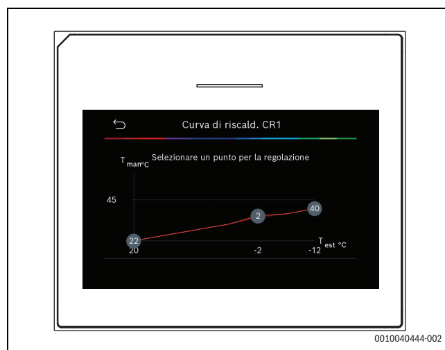
Fig. 1 Schermata iniziale per l'impostazione della curva termocaratteristica di riscaldamento per il tipo di regolazione in funzione della temperatura esterna con punto base (e punto di comfort)
