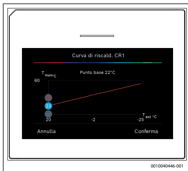
Fig. 3 Regolare il punto base
